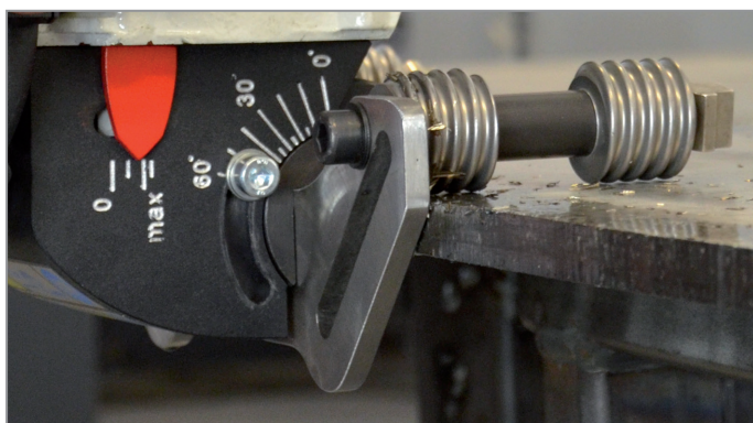
Plynulo nastaviteľný uhol úkosu v rozsahu 0 - 60°
